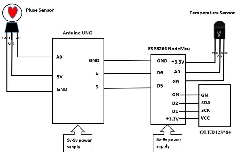
الشكل (3): الرسم التخطيطي للمكونات المادية
