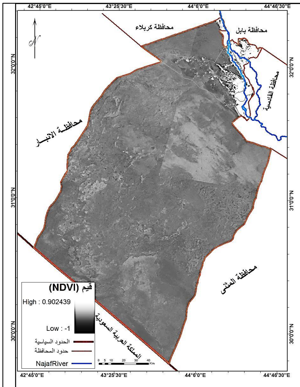
خريطة ( 4 ) قيمة لمؤشر الاختلاف الخضري الطبيعي (NDVI) للعام 1990
