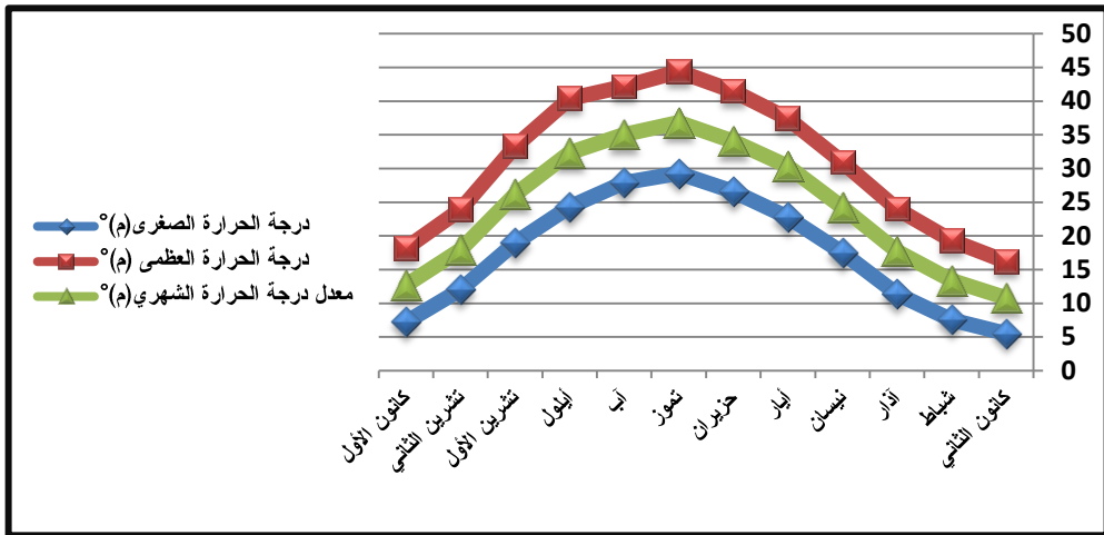
شكل (1) درجات الحرارة العظمى والصغرى والمعدل العام (م) في محافظة النجف
