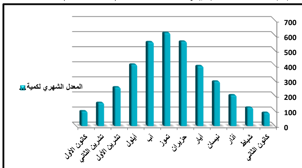
شكل (4) معدلات كمية التبخر (ملم) في محافظة النجف للمدة (1990-2020)
