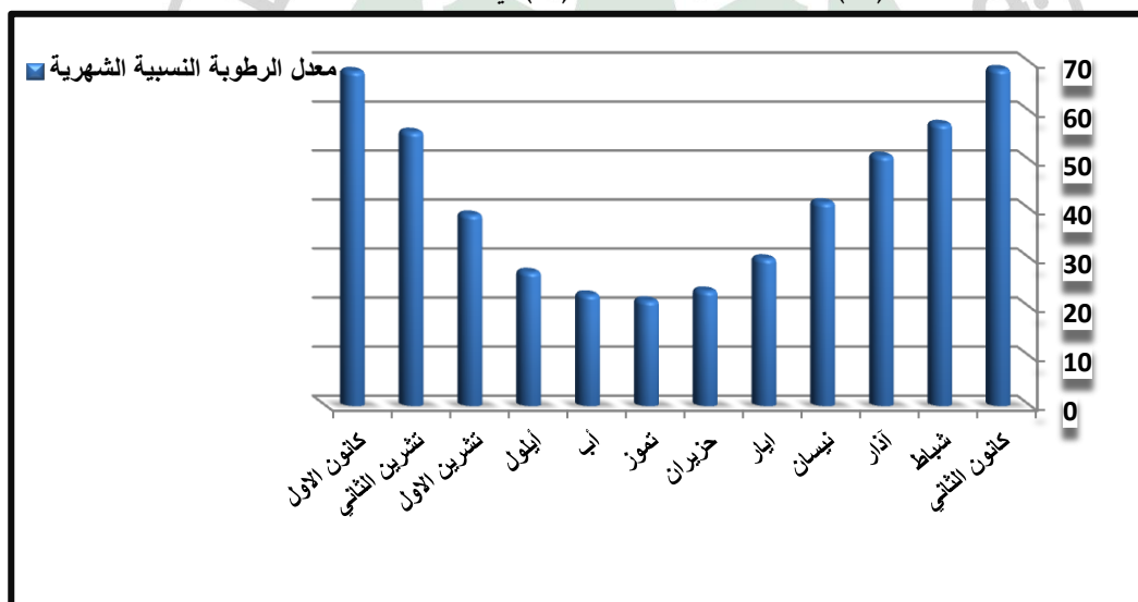
شكل (2) معدلات الرطوبة النسبية (%) في محافظة النجف
