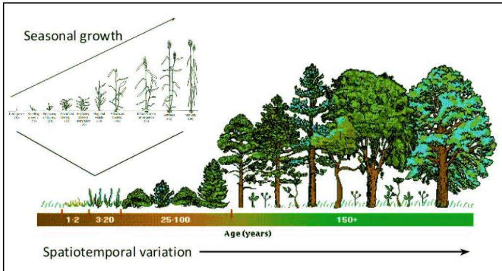
الشكل ( 6 ) النمو الموسمي المرسوم مقابل التباين الزماني المكاني
