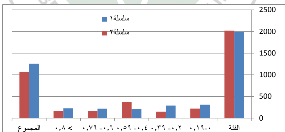
شكل (8) قيم فئات (NDVI) لمحافظة النجف الاشرف للمدة (1990-2020)
