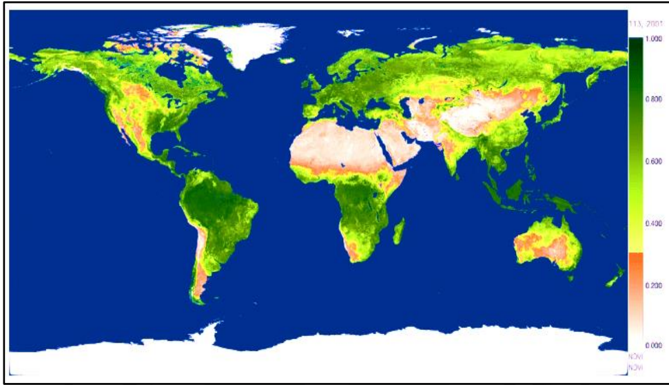
الشكل ( 5 ) مؤشر الاخضرار (NDVI) على مستوى العالم
