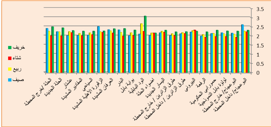
شكل (٤) يوضح قيم عنصر (CH 4 ) ونسبة تواجدته في هواء وبحسب القيم بمحطات الوقود في قضاء الحلة ولأربعة فصول
